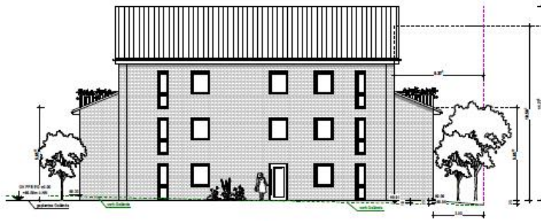
OSTANSICHT Haus 3
