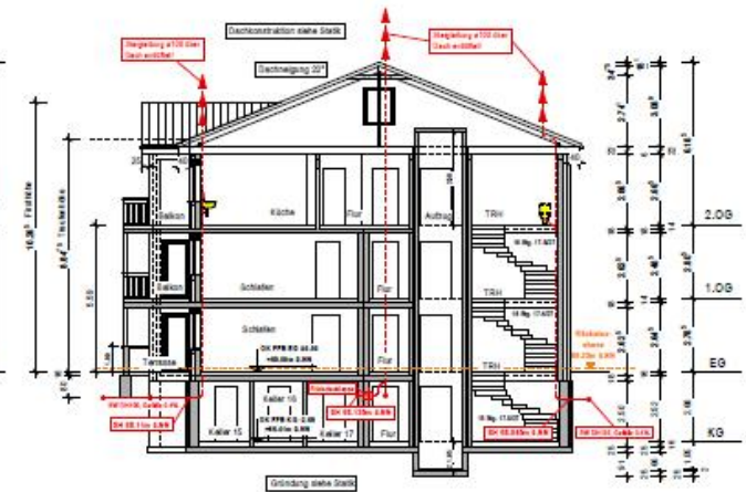
SCHNITT A - A Haus 3
