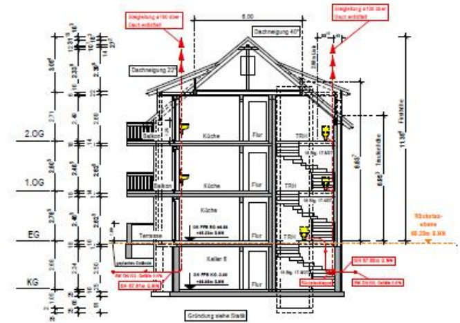
SCHNITT A - A Haus 2
